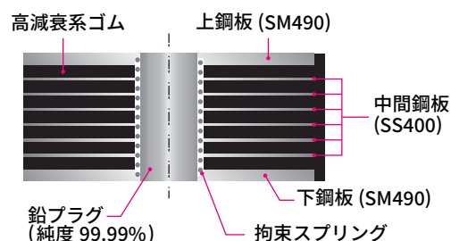
拡大断面図
