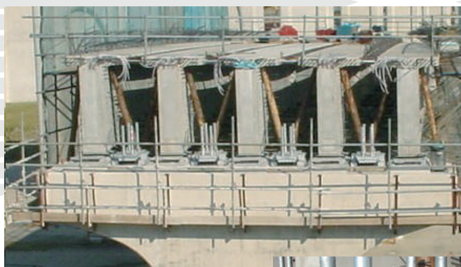
機能分離型支承の実施例
