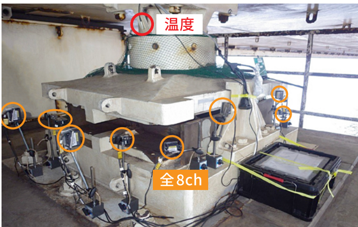
設置状況
